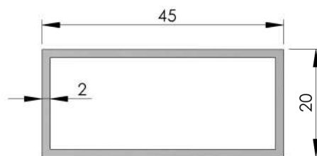
PERFIL 45x20
